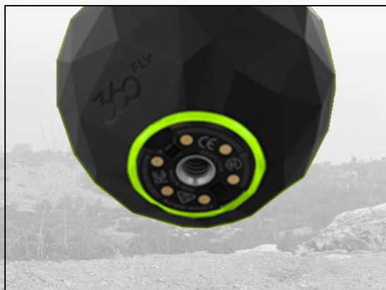
高い互換性を持つ 下部マウント部（1/4-20UNCメス）
